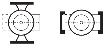
Fig. 1 Orientación recomendada de la caja de conexiones
