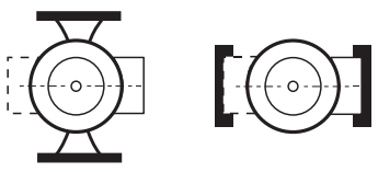
Fig. 1 Orientation recommandée de la boîte à bornes
